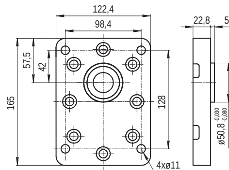
63 EUROPEAN \varnothing 50,8
