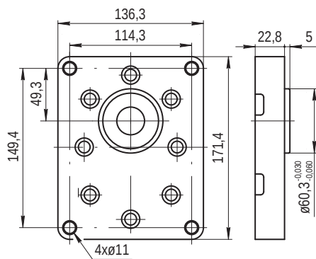
64 EUROPEAN \varnothing 60,3
