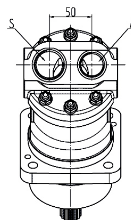
насос левый
