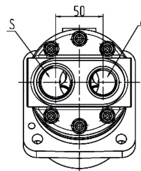
насос левый
