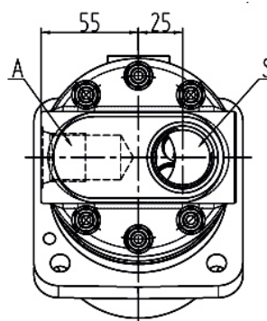
насос правый
