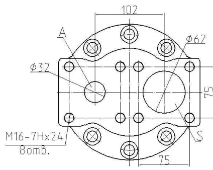
насос правый
