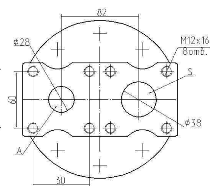
насос правый
