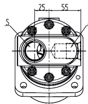
насос левый
