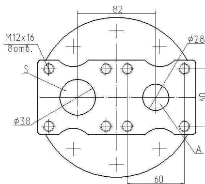
насос левый
