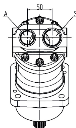
насос правый
