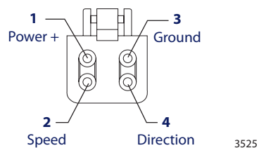
4 pin Deutsch® Plug DT Series Connector
