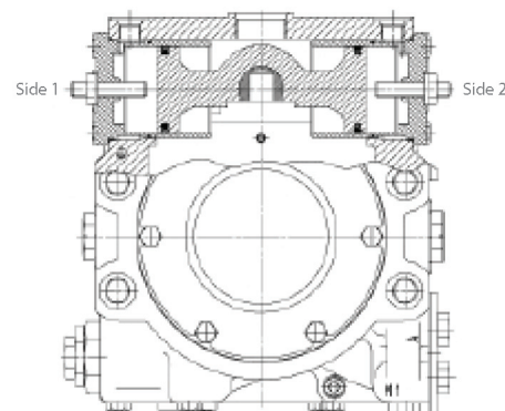
Displacement limiter
